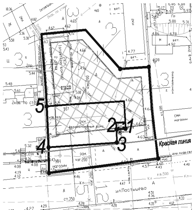
Схема границ земельного участка с кадастровым номером 25:31:010401:695 с отображением места размещения планируемого к реконструкции объекта капитального строительства
